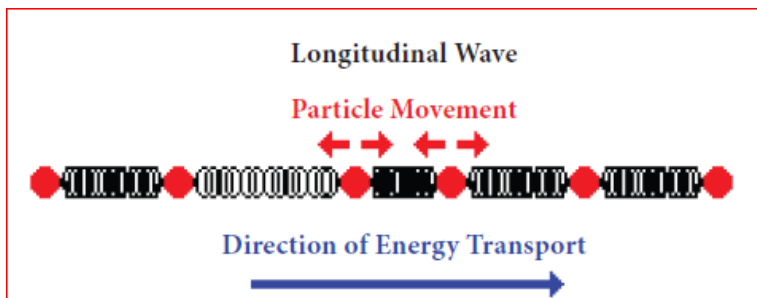
Longitudinal wave
